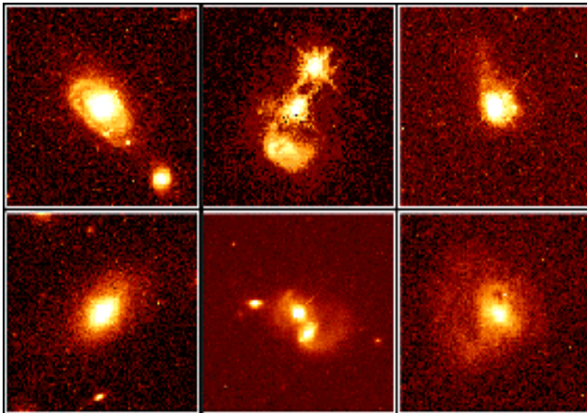
Cuásar cúmulo de galaxias. HST-WFPC2. NASA
