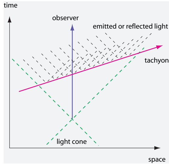
FIGURE 114 Diagrama espacio-tiempo de una hipotética observación de un taquión.
