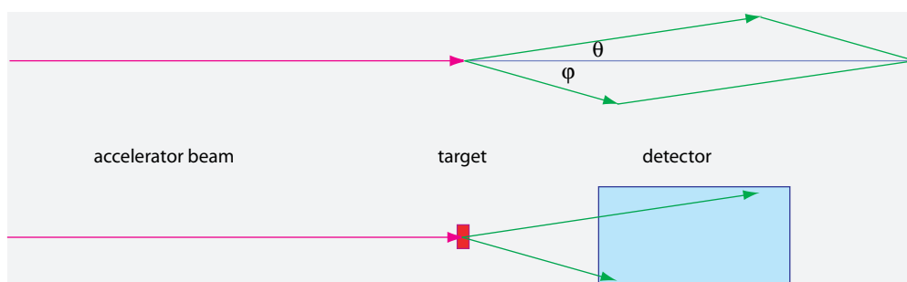
FIGURE 118 Las dimensiones de los detectores en los aceleradores de partículas se basan en la regla de ángulos del billar relativista.
