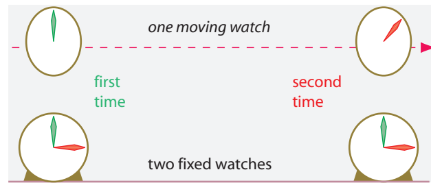
FIGURE 93 Los relojes en movimiento se atrasan
