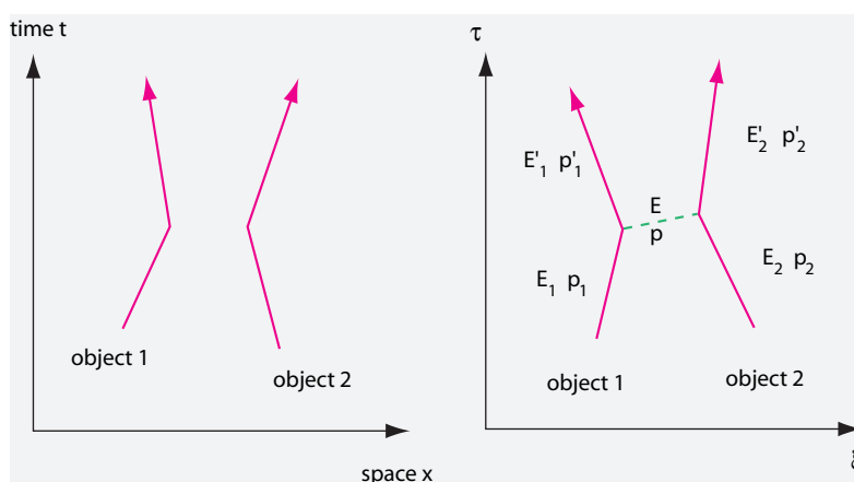
FIGURE 119 Diagrama espacio-tiempo de una colisión para dos observadores.
