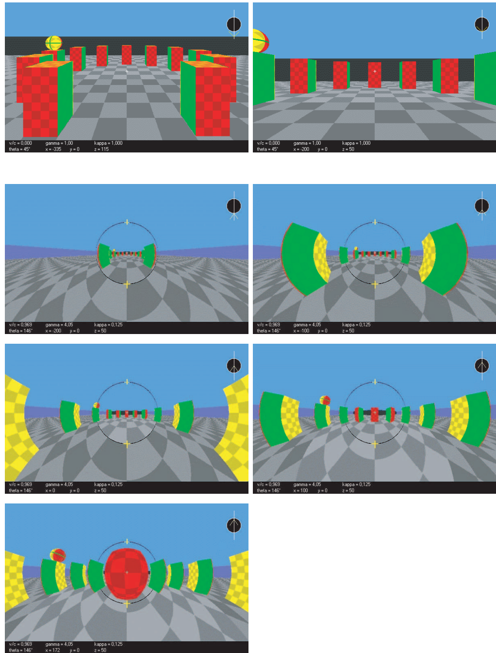
FIGURE 108 Vuelo a través de doce columnas verticales (mostradas en las dos imágenes de arriba) a una velocidad 0.9 veces la de la luz, según Nicolai Mokros and Norbert Dragon, que muestra el efecto de la velocidad y la posición en las distorsiones (© Nicolai Mokros)
